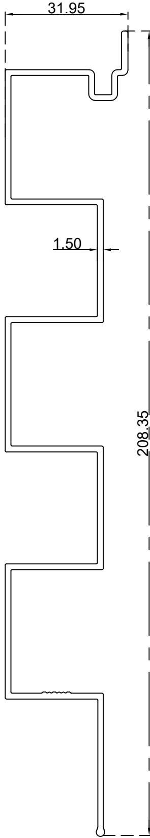
غطاء جدار 221.17 ملم الرقم التسلسلي للصف: BLT3551 الوزن 1.513:(Kg/m)
